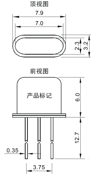
单位: mm, 公差: ±0.20mm
