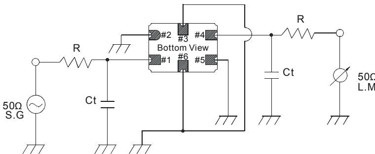
晶体滤波器测试线路图(3Poles)
