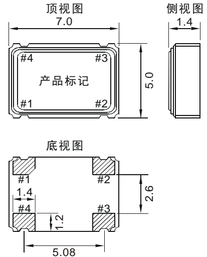
单位: mm, 公差: ±0.20mm
