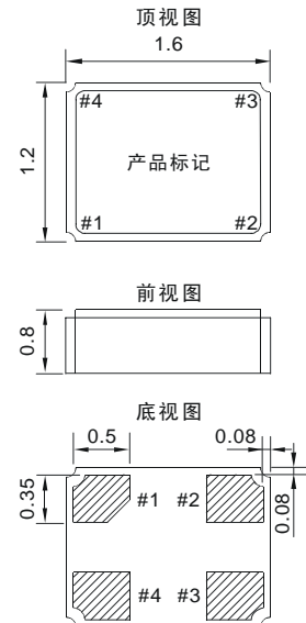
单位: mm, 公差: ±0.20mm
