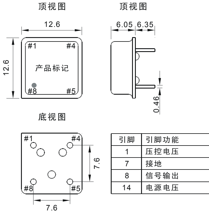
封装尺寸:
